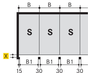
Garages alignés avec portes simples (respectivement 2 voitures)
