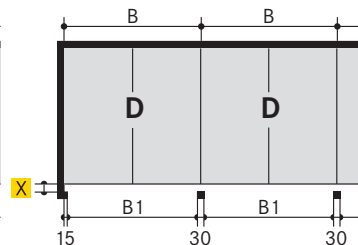
Garages alignés avec portes doubles (respectivement 4 voitures)
