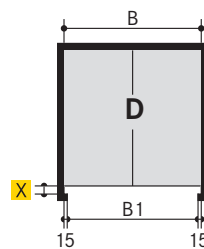
Garages alignés avec portes doubles (respectivement 4 voitures)
