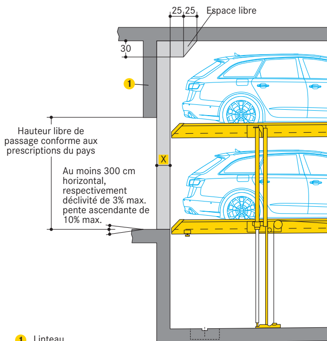
Installation simple (2 voitures)
